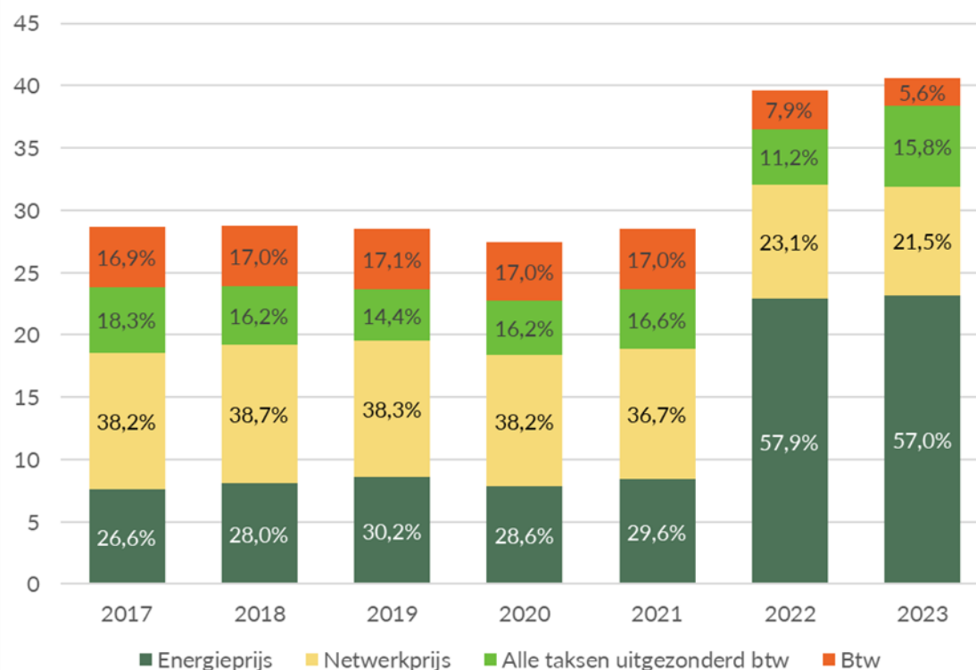
Figuur 12: Electriciteitsprijs verloop in eurocent/kWh (consumptieblok DC – 2500 tot 5000 kWh/jaar)
