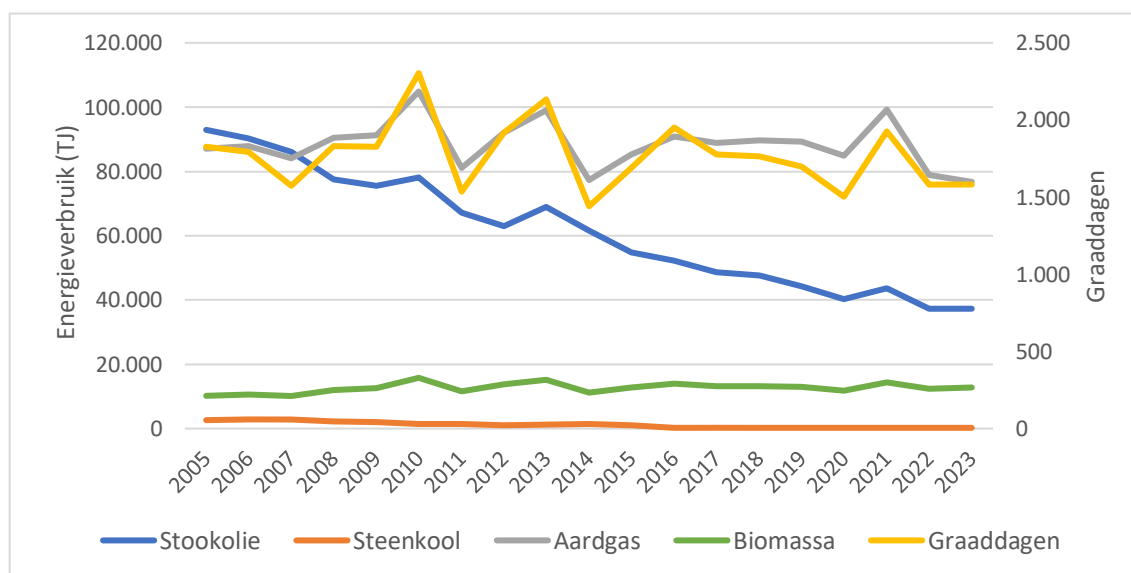
Figuur. Evolutie energieverbruik per brandstoftype residentiële sector (excl. offroad) 2005-2023
