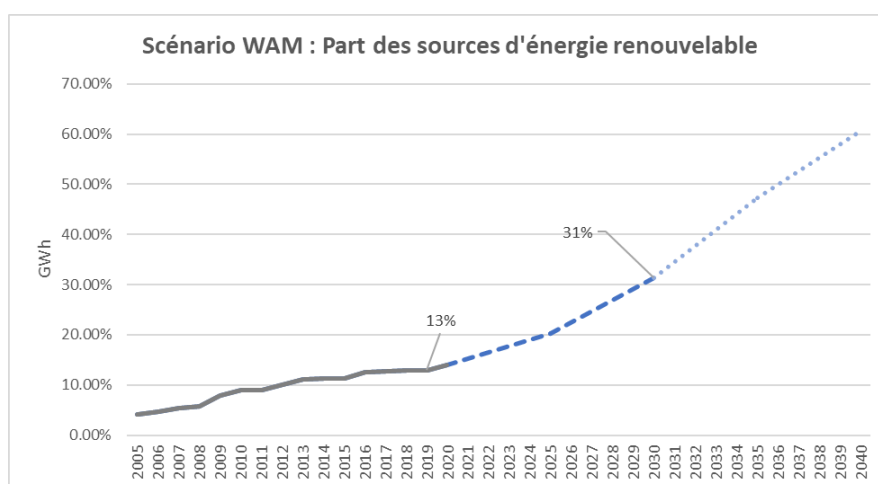
Afbeelding. Evolutie van het aandeel hernieuwbare energie in Wallonië in het scenario met bijkomende maatregelen ('WAM') (2005-2040), 2002-2020: energiebalans; 2021-2040: resultaten van het TIMES-model
