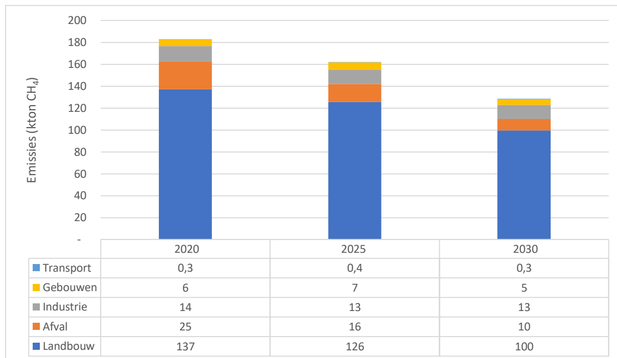
Figuur. Methaanprognoses WAM-scenario 2020-2030
