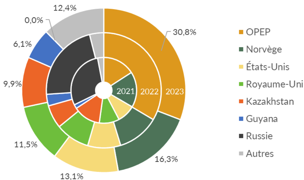
Figuur. Oorsprong van invoer van ruwe olie
