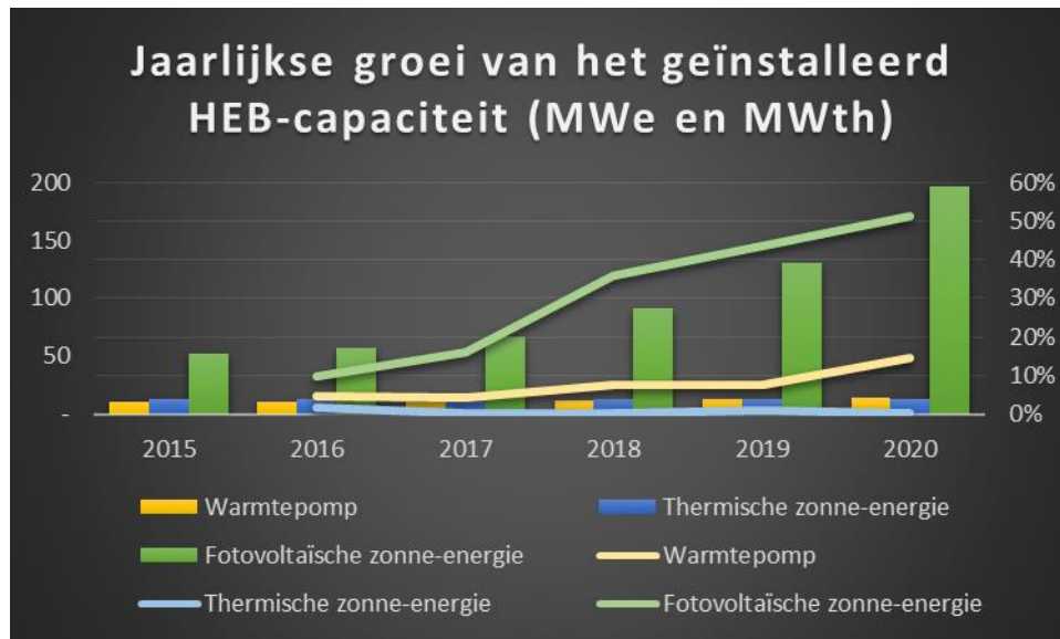
Figuur. Geïnstalleerde capaciteit van hernieuwbare energie in Brussel 2015-2020 (Bron: RENAQ).
