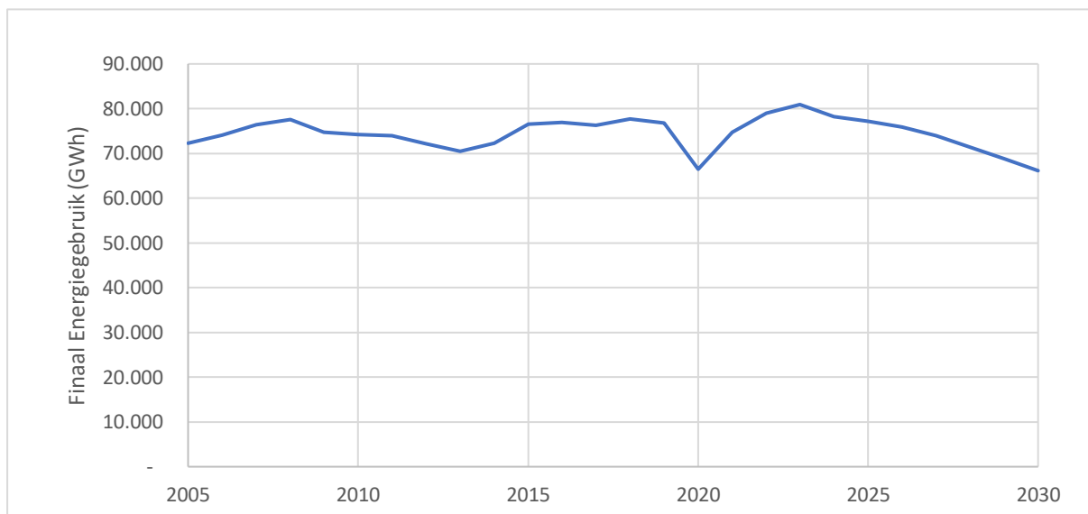
Figuur. Evolutie finaal energiegebruik transport 2005-2030 (in GWh)
