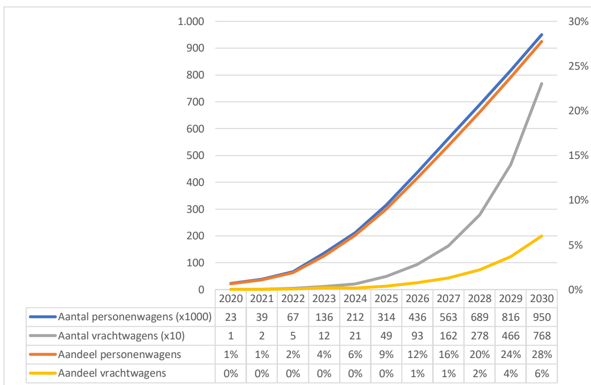
Figuur. Evolutie zero-emissie personen- en vrachtwagens in totale vloot (aantallen en aandelen) in de periode 2020-2030
