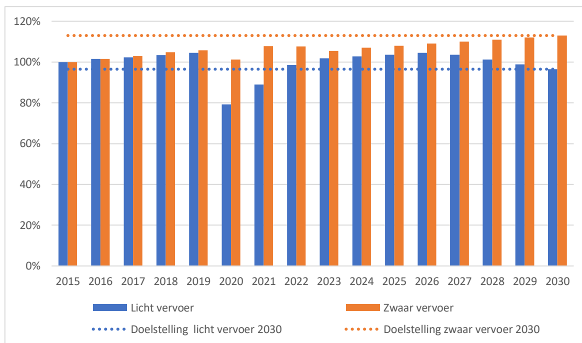
Figuur. Evolutie voertuigkilometers zwaar en licht vervoer in de periode 2015-2030 in het WAM-scenario (uitgedrukt in % t.o.v. 2015) (2024-2030 = prognoses)
